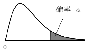
図1 \chi^2 分布
