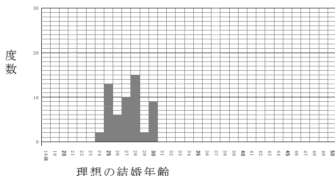
図1 母集団における全数調査の分布
