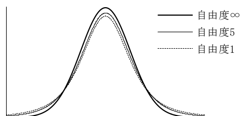
図1 自由度1、5、∞のt分布
