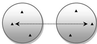
完全連結 [最遠接法]
